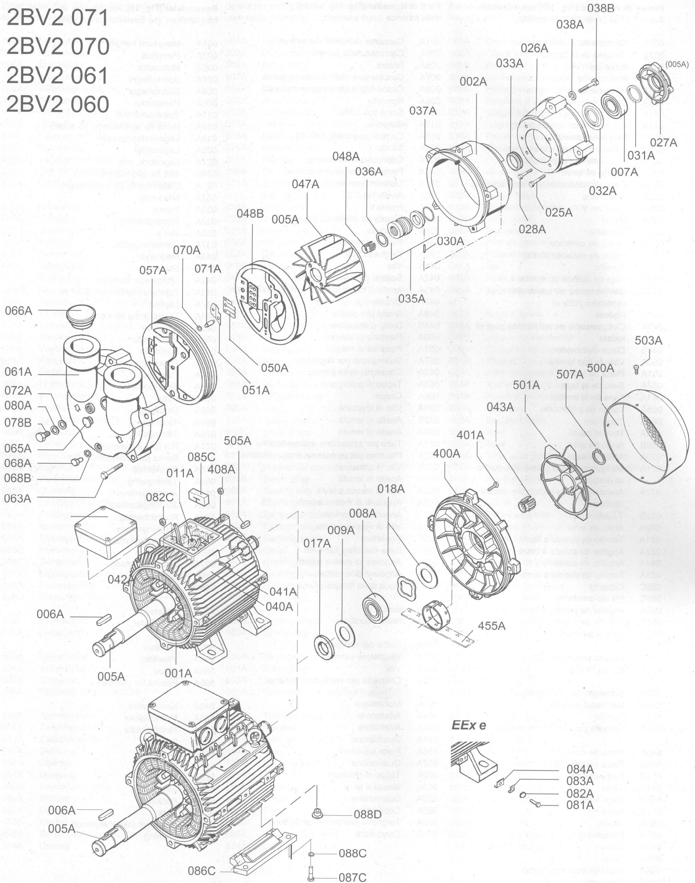
Fig. 16 Darstellung einer zerlegten 2BV2-Vakuumpumpe/-Kompressor Exploded view of a 2BV2 vacuum pump/compressor Pompe à vide/compresseur 2BV2 en vue éclatée Representación de una bomba de vacío/compresor 2BV2 despiezados Rappresentazione di una pompa per vuoto/un compressore 2BV2 smontato Sprängskiss av isärtagen vakuumpump/-kompressor 2BV2
